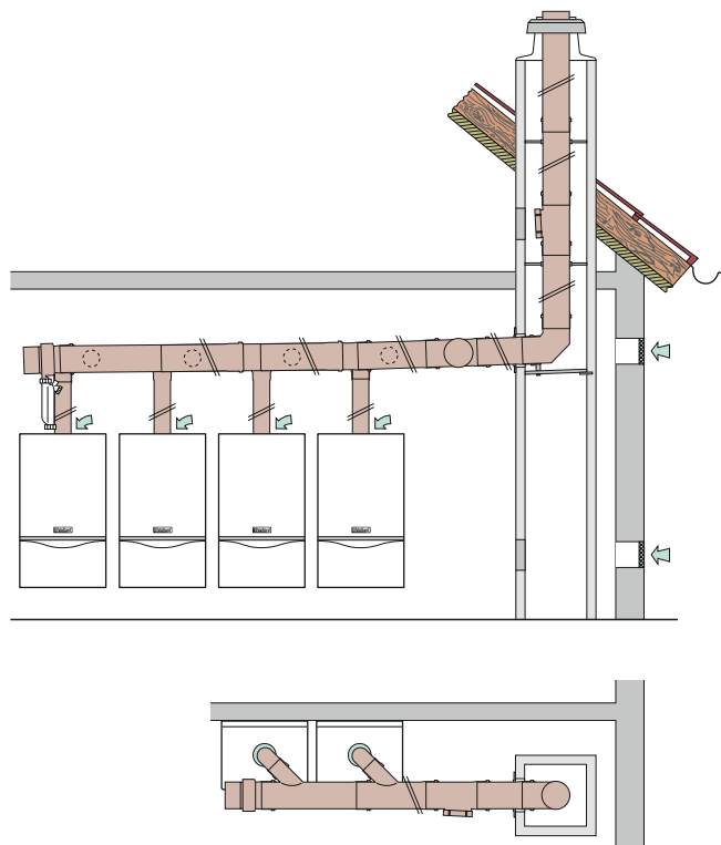
Sistem kaskadnog dimovoda, kod kaskadnog spajanja uređaja
