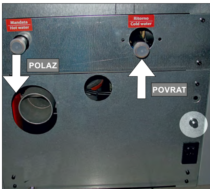
Slika 5. Polaz, povrat
