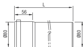
PP nastavak (L = 500-1000-2000 mm)
