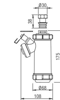
PP sifon
