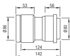
Kruto - fleksibilni spoj F od PP
