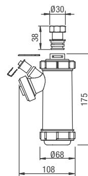
PP sifon
