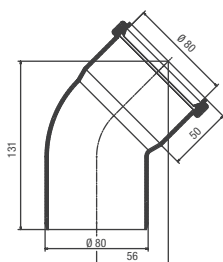
Koleno 45°
