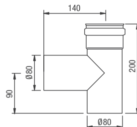
"T" element za povezivanje
